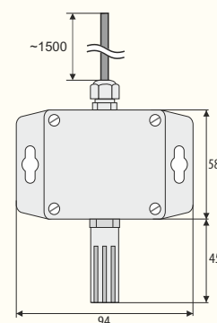
Sonda zewnętrzna z przewodem AR253/2
