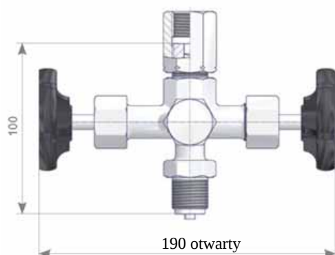
Zawór z przylączem testowym M 20 x 1,5
