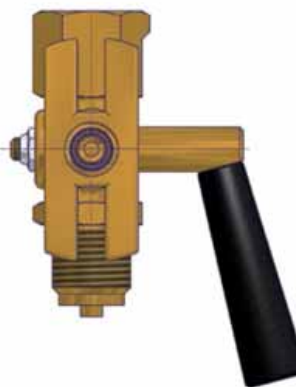
Kurek manometryczny z kołnierzem testowym 60 \times 25 \times 10
